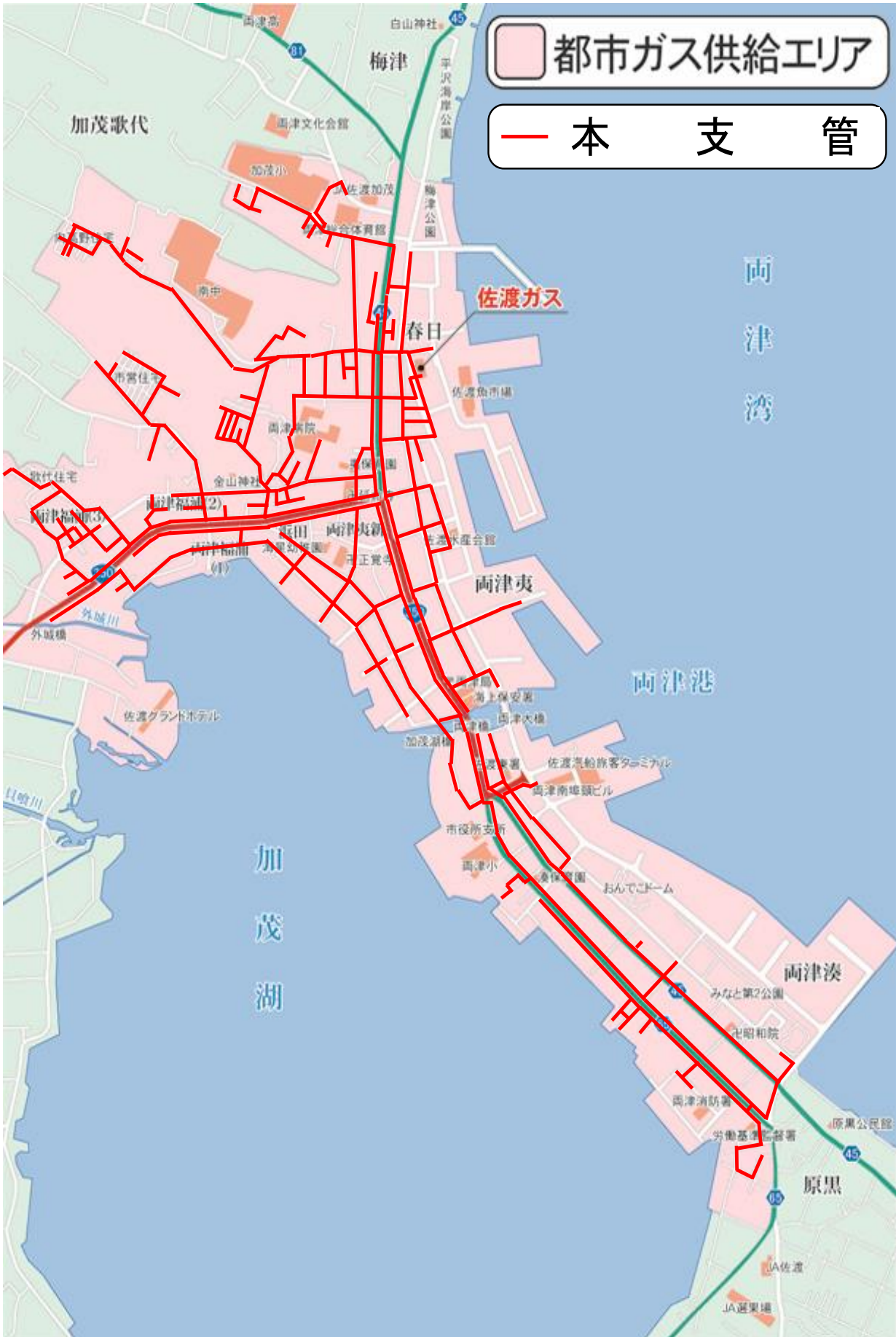
(導管)第7表 供給計画図(第8表を兼ねる)
